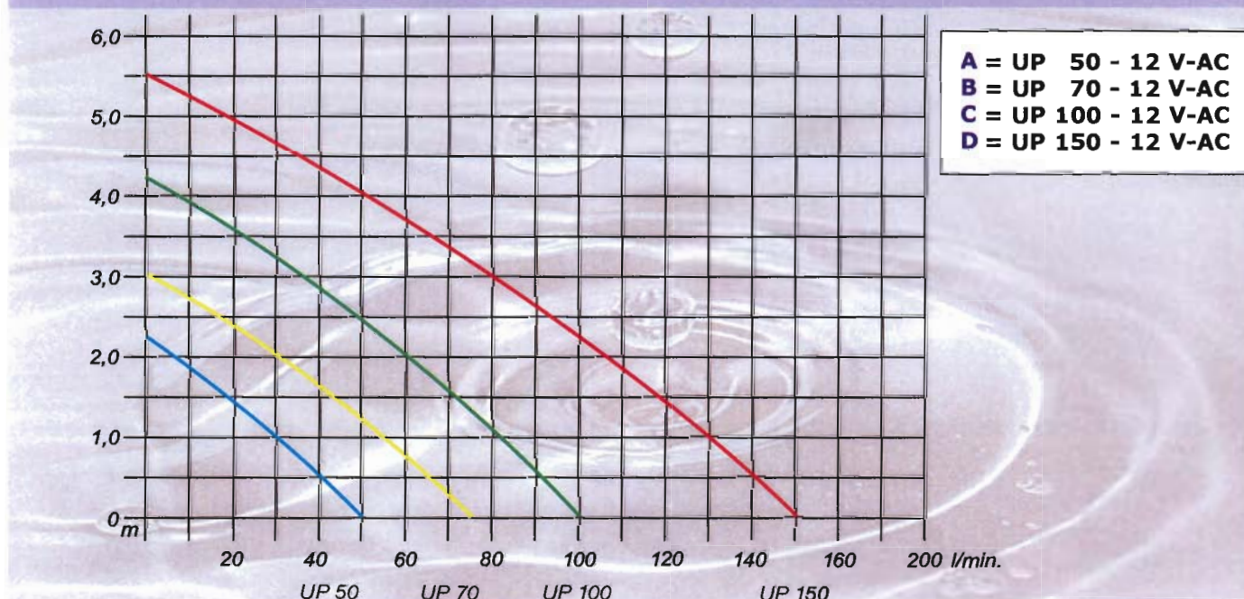
Leistungsdiagramm Niedervoltpumpen Typ UP 12 V-AC
