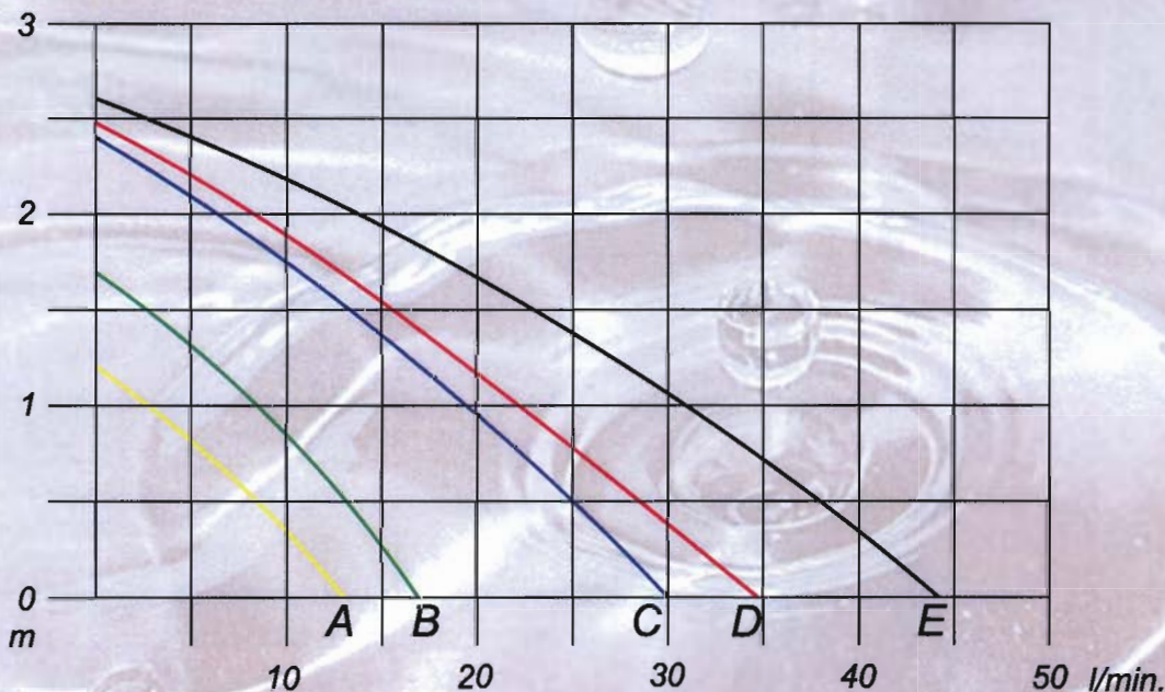
Leistungsdiagramm Pumpentyp UP 10 S, 20 S, 30 MH, 30 S, 40 MH
